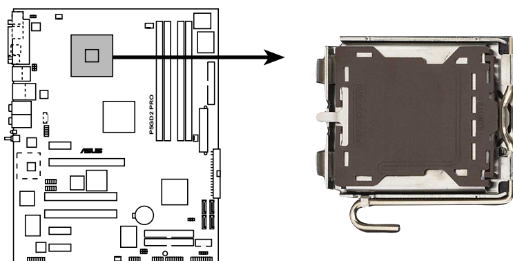
P5GD2 PRO Socket 775
