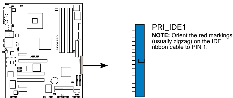
P5GD2 PRO IDE connectors
